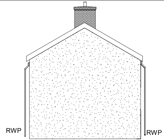
2 East 1 : 100
