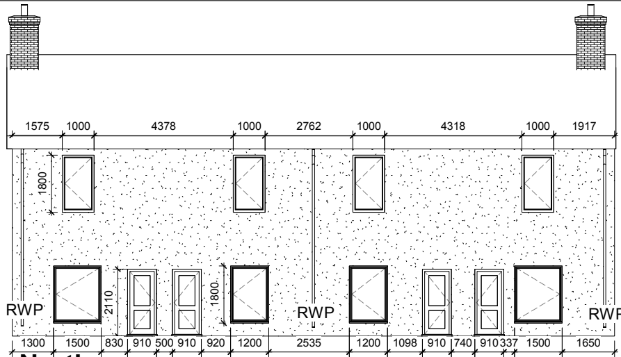
1 North 1 : 100
