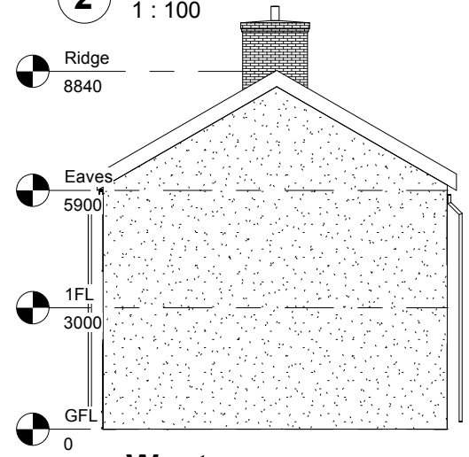
4 West 1 : 100
