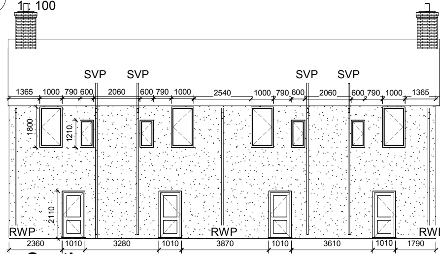
3 South 1 : 100
